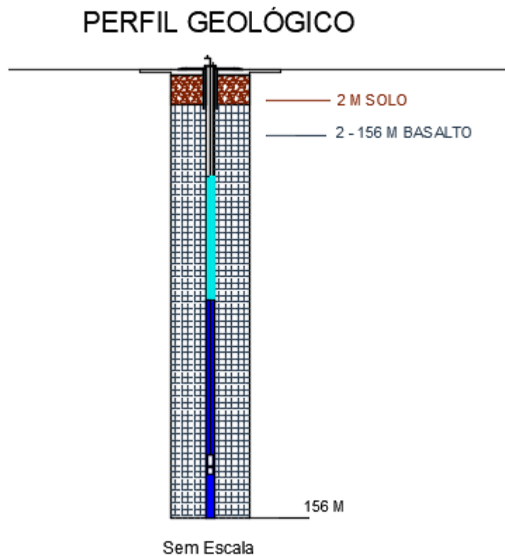
Figura 12: Perfil Geológico do Poço. Fonte: Autor (2023).
