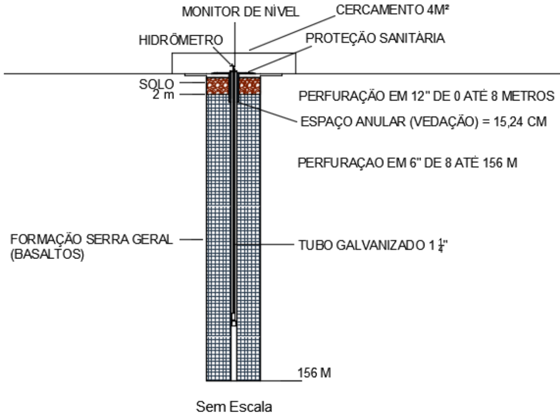
Figura 13: Perfil Construtivo do Poço. Fonte: Autor (2023).
